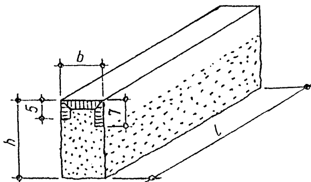
Rys. 5. Obrzeże kamienne
