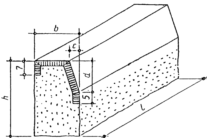
Kształt krawężników ulicznych
